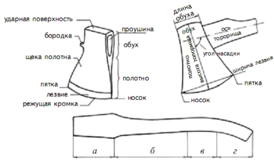
Рис. 112. Травмообразующие детали топора и топорика (по П.В. Скляр, 1960): а — захватывающая часть; б — средняя часть; в — захватная часть; г — хвост
